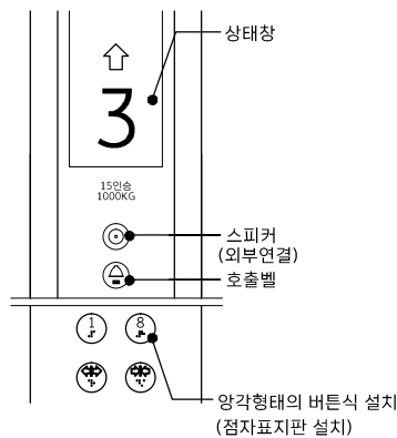
일반조작반
