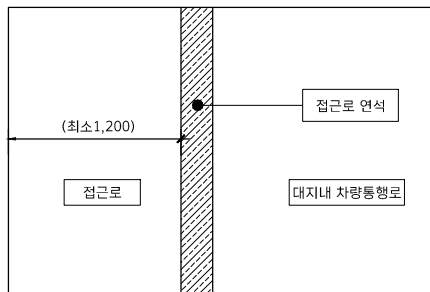
접근로 경계석
