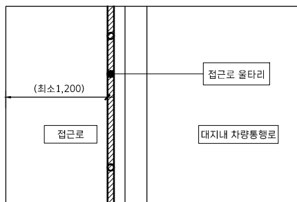
접근로 울타리
