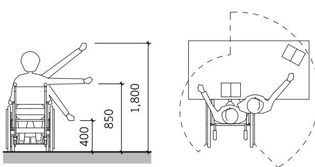
도달치수
