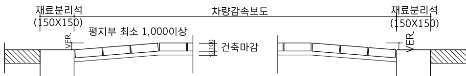
차량감속보도 종단면도
