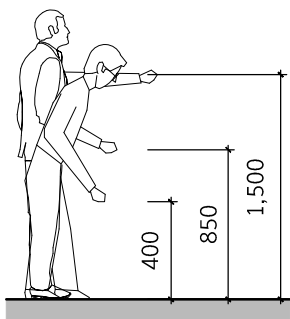
마감치수(유효치수)
