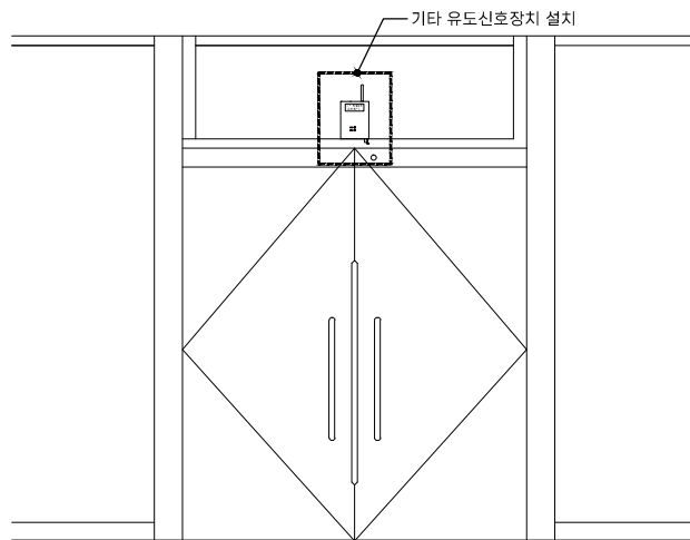
유도신호장치 설치위치-주출입구
